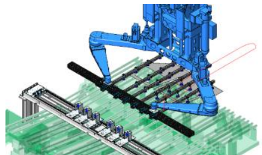
図11 高性能プレス機へキサローダ (株)エイチアンドエフのご厚意による)
