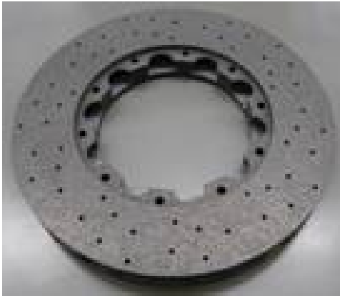
図 20 CMC ブレーキと内部構造（炭素繊維が SiC 化しておらず高強度を維持 13) ）
