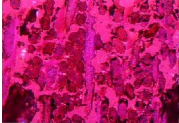
図 20 CMC ブレーキと内部構造（炭素繊維が SiC 化しておらず高強度を維持 13) ）
