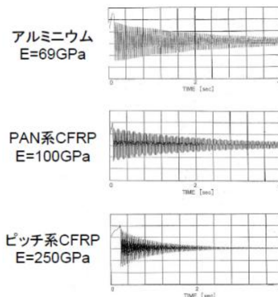
図8 各種材料の振動減衰挙動
