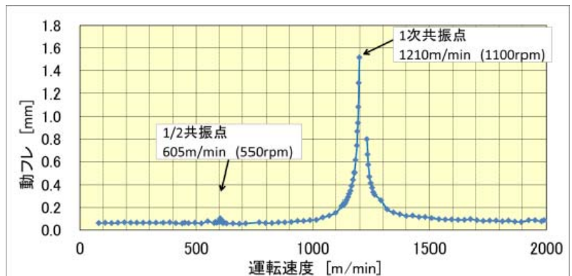
図 13 \phi 350 \times 9,200\text{mmL} ロール 動フレ測定結果
