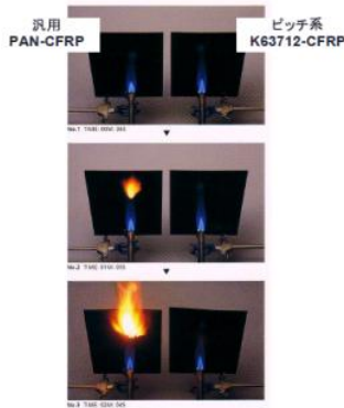
図 17 CFRP 板燃焼試験結果
